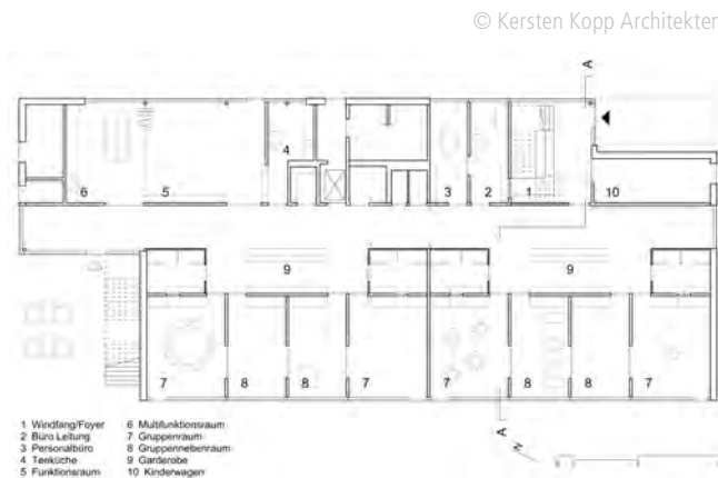
Abb. 3: Beispielhafte Raumanordnung für das Erdgeschoss eines MOKIB
