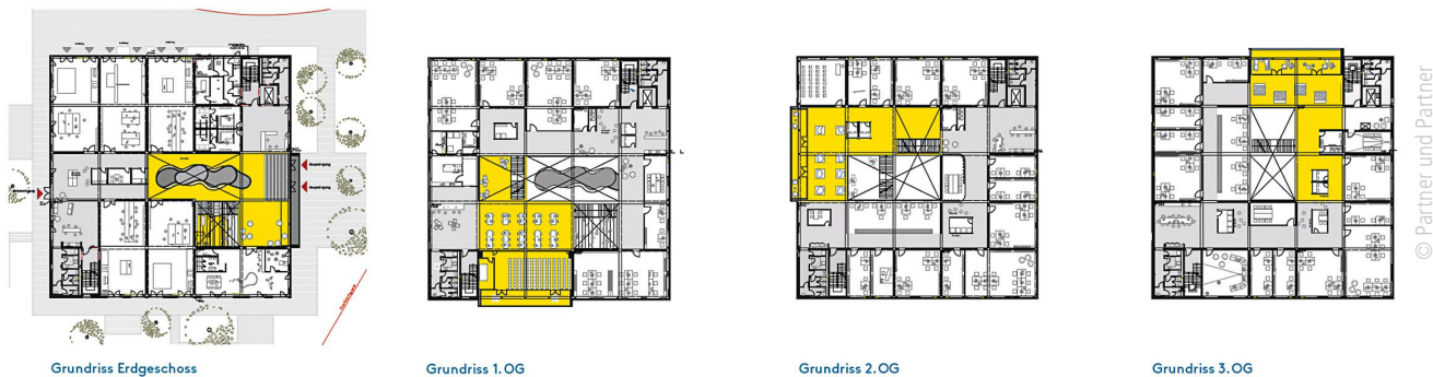
Abb. 4: Grundrisse Gründerzentrum
